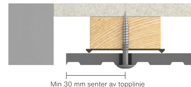
Fig 4. Swisspearl Patina Inline montering av formatkappede plater.
