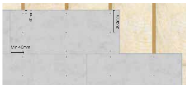
Kantafstande ved standardsamlinger
