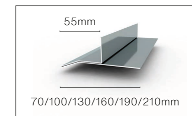
Alu horizontaal raamprofiel Lengte 3000 mm. Verkrijgbaar in alle kleuren. Toepassing: bovenzijde raamkozijn.
