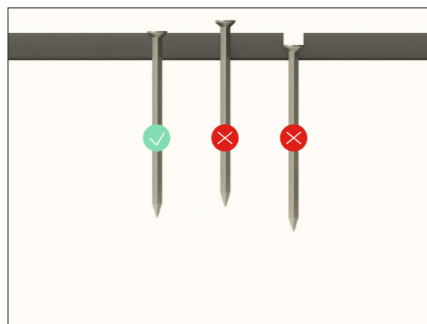
Het bevestigingsmateriaal moet gelijk met het oppervlak van de plank liggen. Geen verzinkboren gebruiken.
