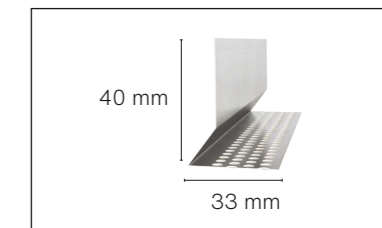
Alu ventilatie startprofiel Lengte 3000 mm. Verkrijgbaar in brut aluminium. Andere kleuren op aanvraag.
