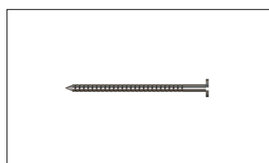
Ringnagels Verkrijgbaar op band in 2,9 x 40 mm en 2,9 x 50 mm in blank RVS en op kleur. Toepassing: nagelen Swisspearl Plank.
