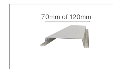
Geventileerd omega-profiel Lengte 3000 mm. Verkrijgbaar in thermisch verzinkt staal. Toepassing: enkel horizontaal regelwerk bij verticale toepassing Swisspearl Plank.
