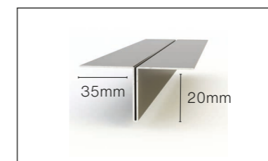
Alu verticaal T-profiel Lengte 3000 mm. Verkrijgbaar in alle kleuren.
