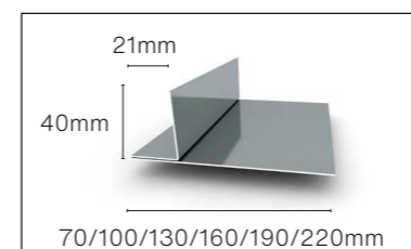
Alu verticaal raamprofiel Lengte 3000 mm. Verkrijgbaar in alle kleuren. Toepassing: zijkant raamkozijn.
