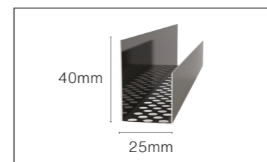
Geventileerd U-profiel Lengte 3000 mm. Verkrijgbaar in thermisch verzinkt staal. Toepassing: boven en onderin gevel bij verticale toepassing Swisspearl Plank.
