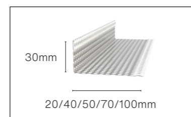
Alu ventilatieprofiel Lengte 3000 mm. Verkrijgbaar in brut aluminium. Andere kleuren op aanvraag.
