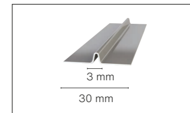
Alu voegprofiel Lengte 3000 mm. Verkrijgbaar in zwart. Andere kleuren op aanvraag.
