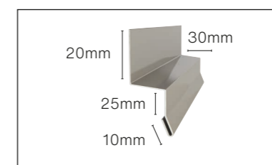
Alu waterslagprofiel Lengte 3000 mm. Verkrijgbaar in alle kleuren.
