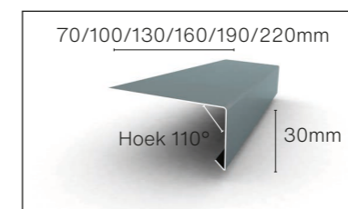
Alu raamdorpelprofiel Lengte 3000 mm. Verkrijgbaar in alle kleuren. Toepassing: onderzijde raamkozijn.
