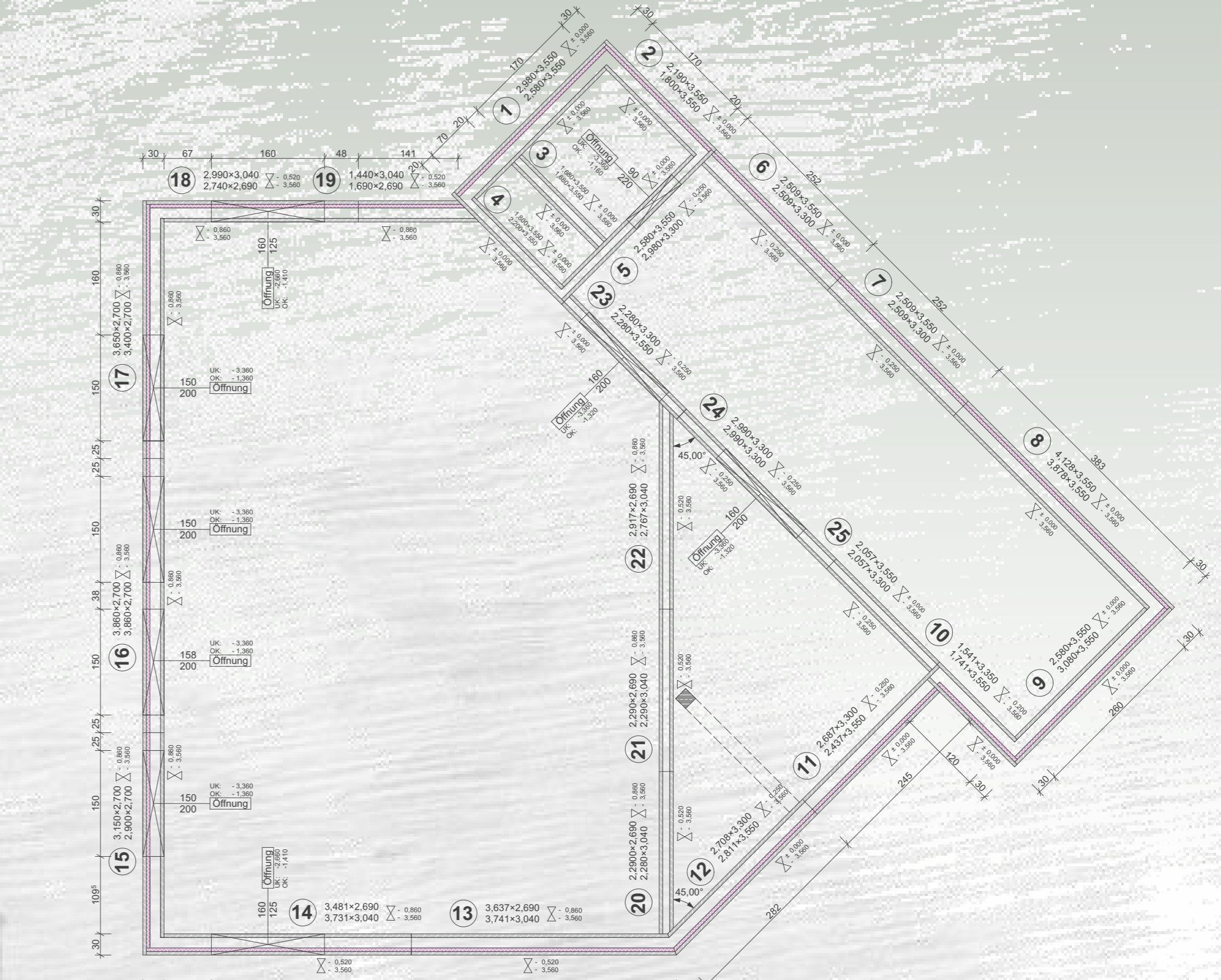
VERLEGEPLAN HOHLWÄNDE UG
