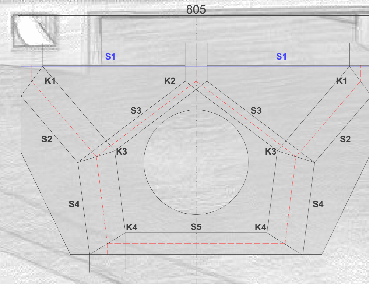
FACHWERKMODELL WANDSCHEIBE
