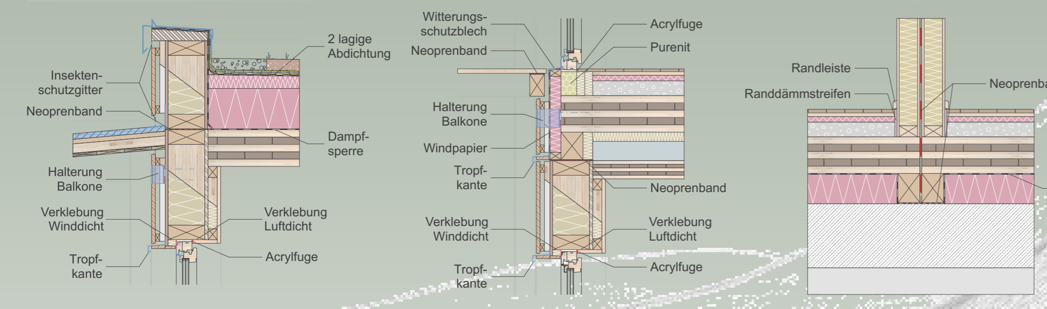
DETAILE HOLZBAU
