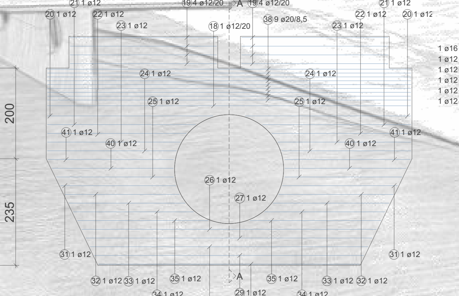
BEWEHRUNG HINTEN HORIZONTAL
