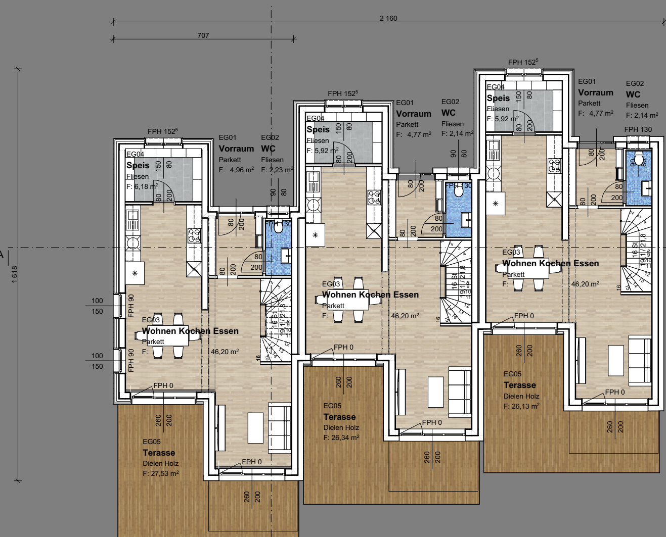
Grundriss Erdgeschoss
