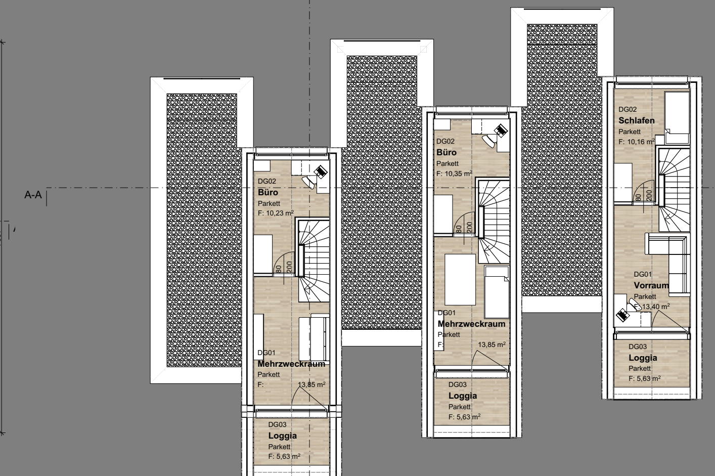
Grundriss Dachgeschoß
