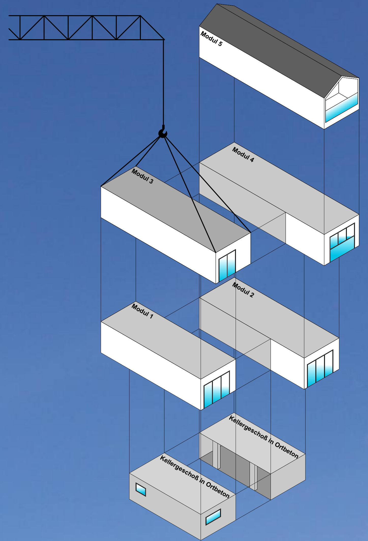
Explosionszeichnung
