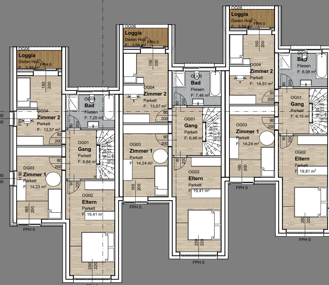
Grundriss Obergeschoß
