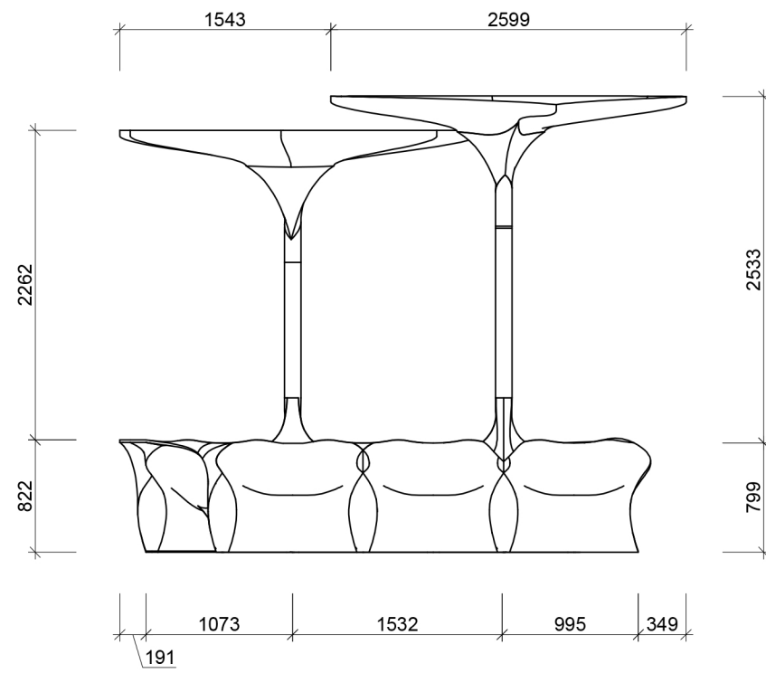
AUFRISS
