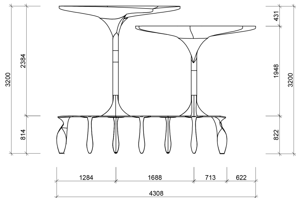
AUFRISS
