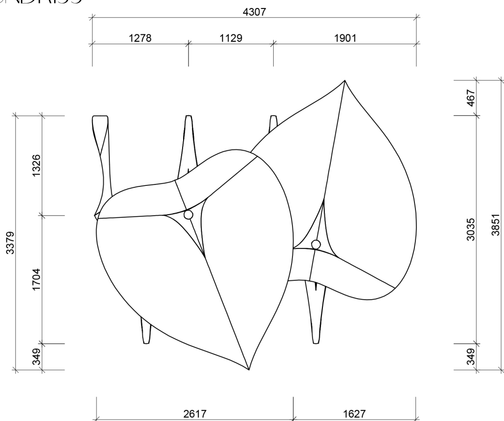
GRUNDRISS
