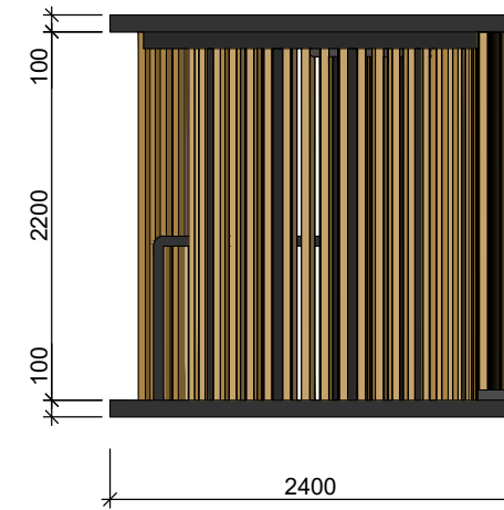
Kreuzriss v.l. M 1:50
