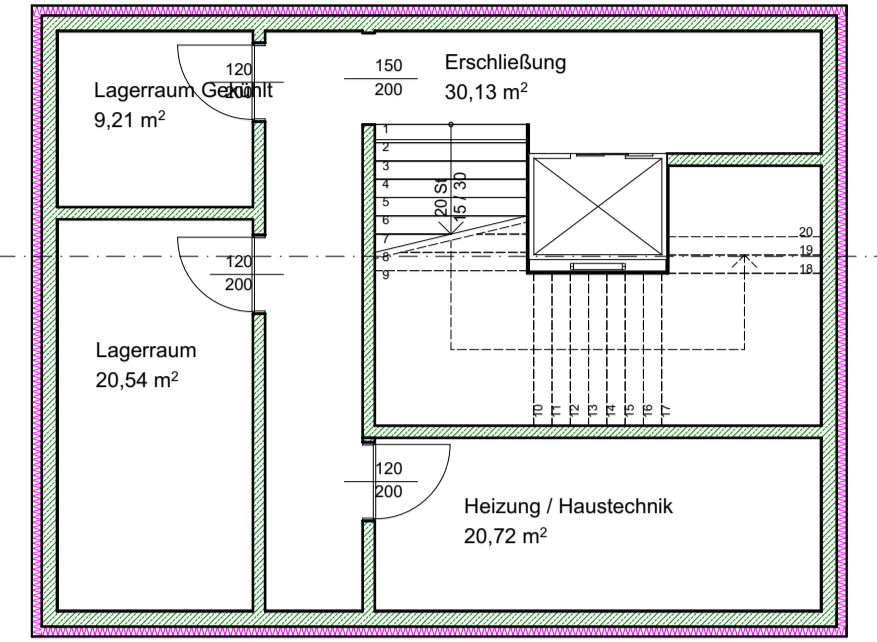
Keller
