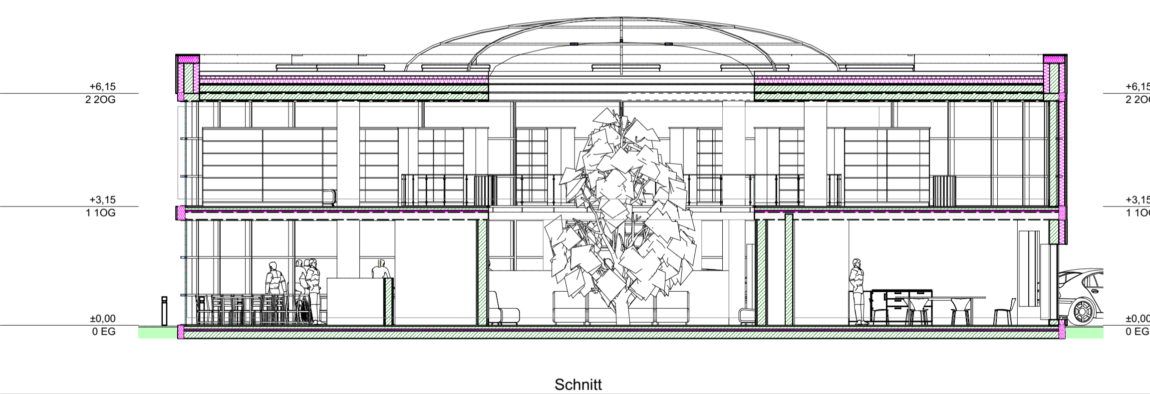
Schnitt
