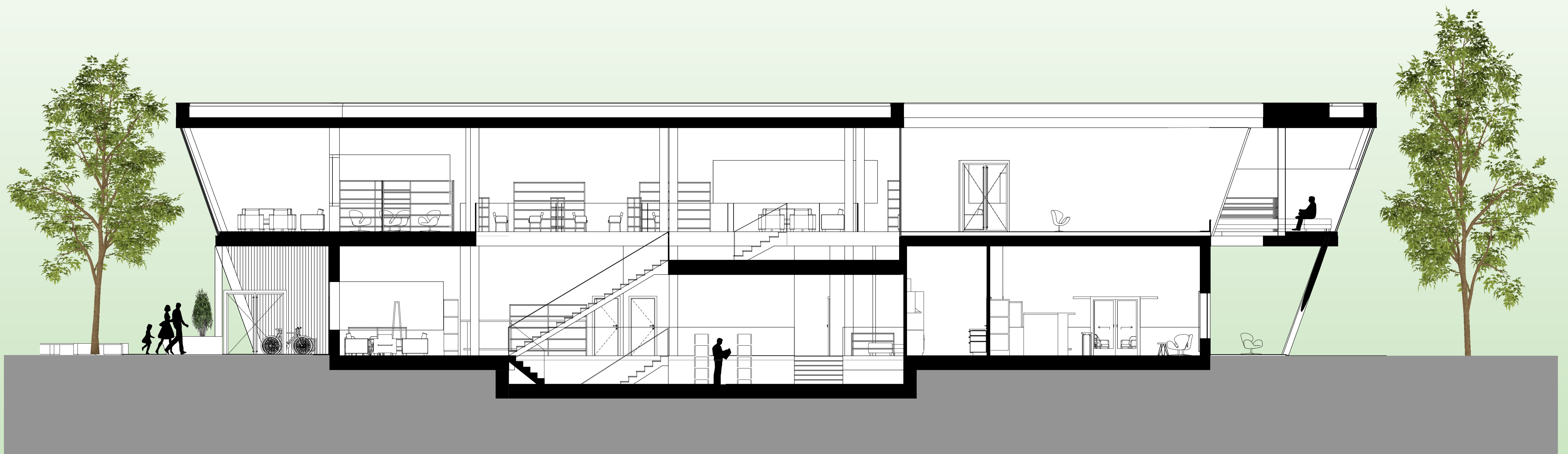
SCHNITT M1:100
