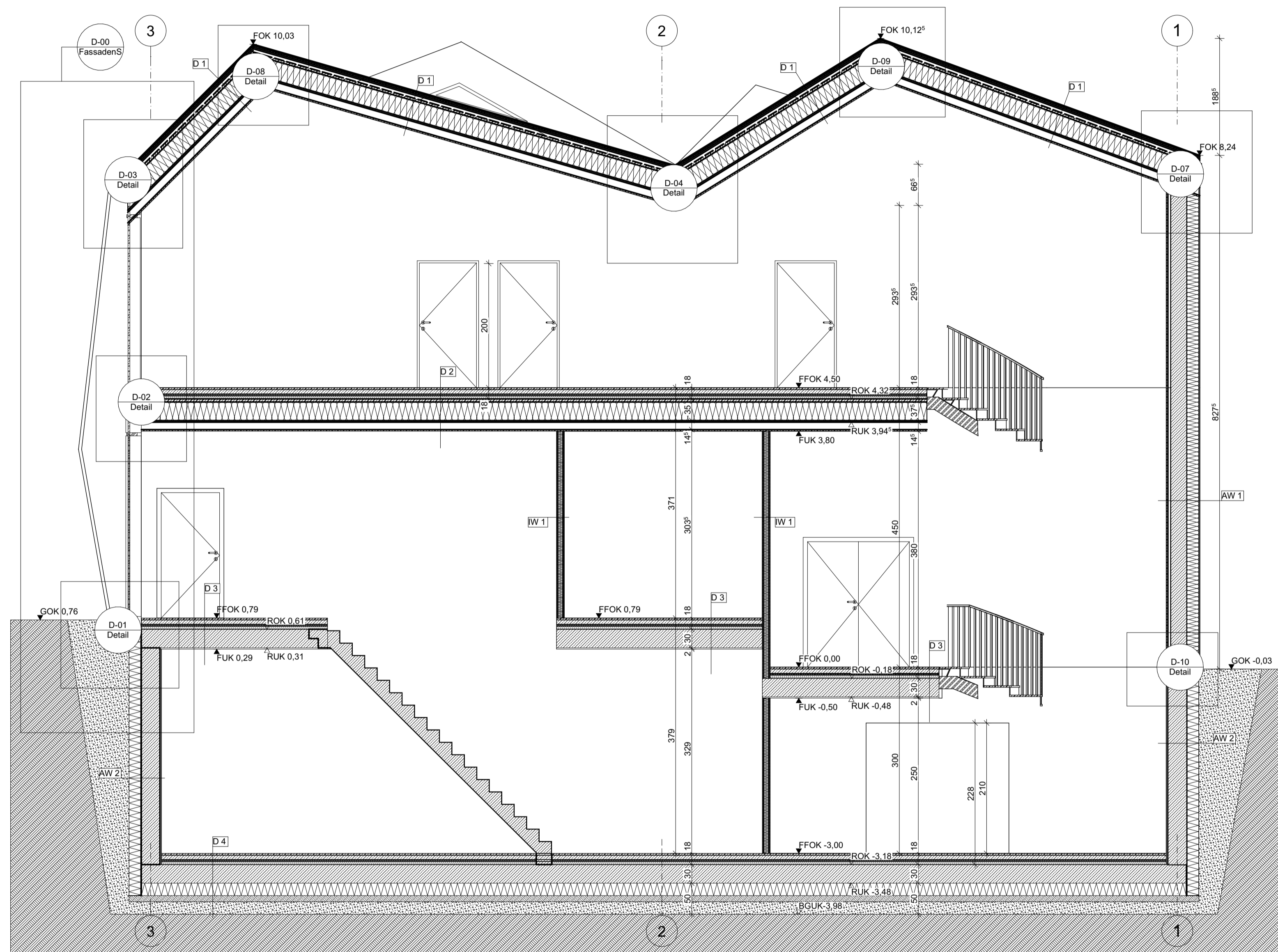
Schnitt 1-1 M 1:50
