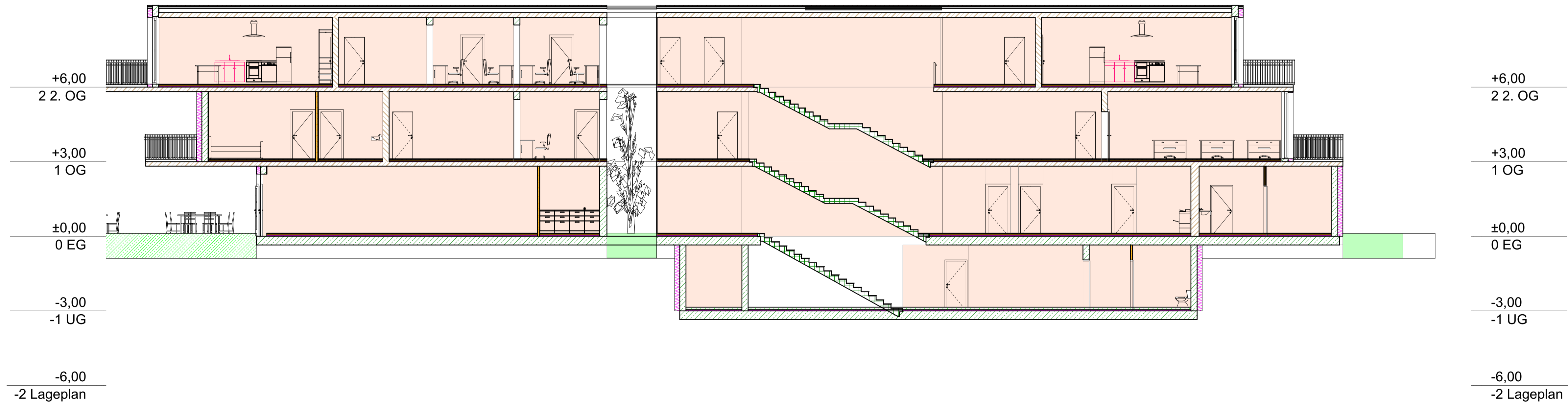
Schnitt (2)
