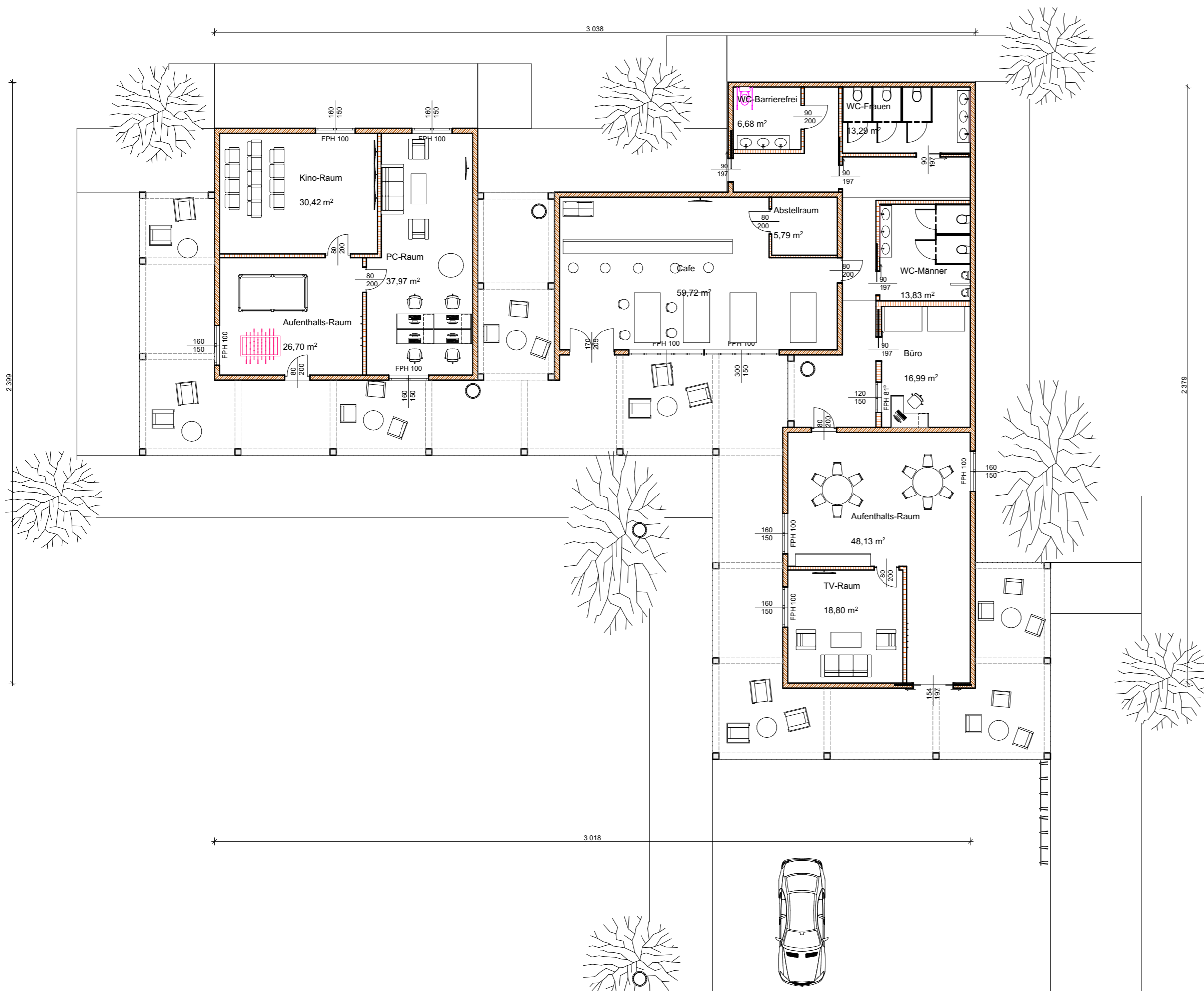
GRUNDRISS
