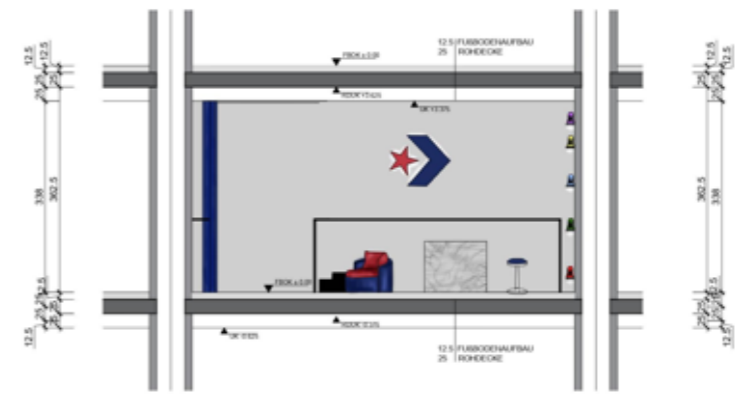
SCHNITT B
