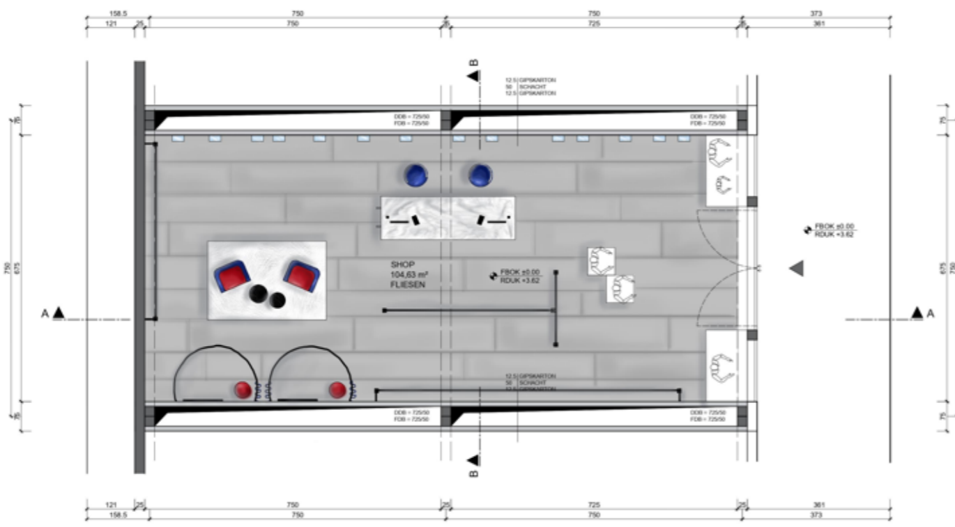
GRUNDRISS
