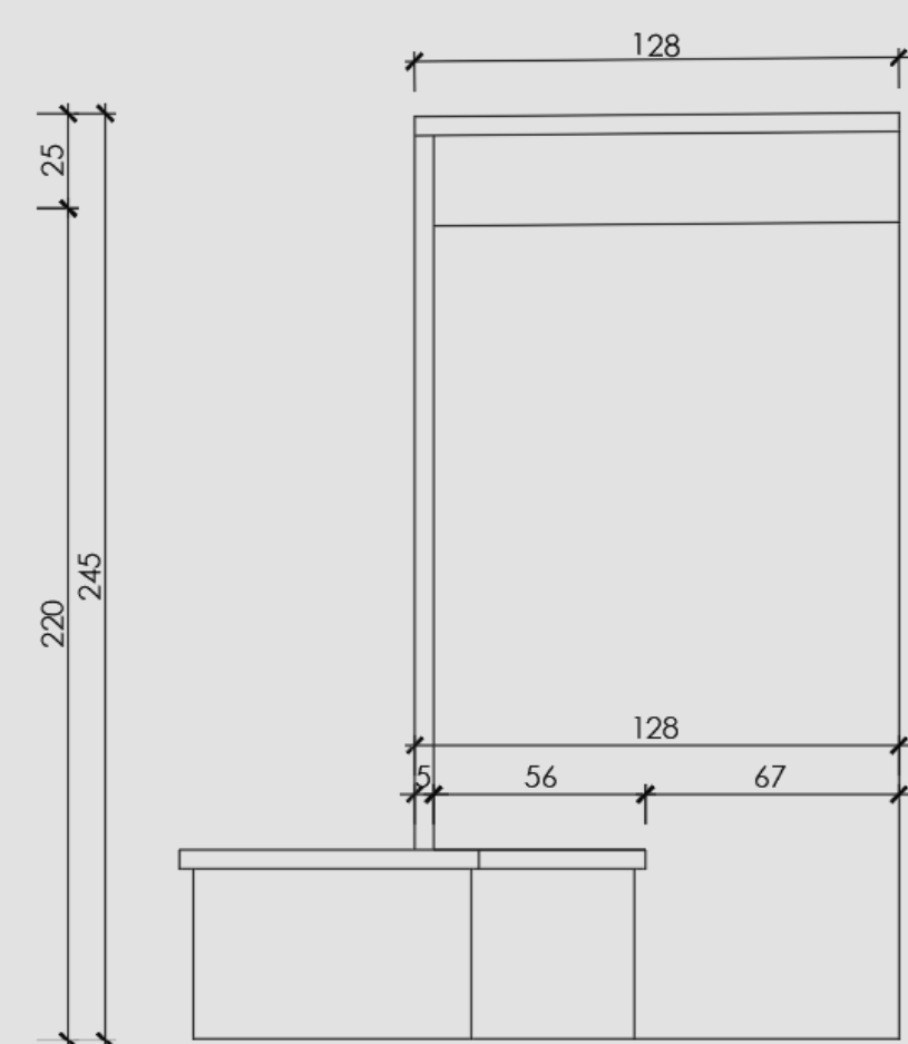
KREUZRISS
