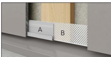
Bild 7 A. Swisspearl Plank Connect Anfangsprofil B. Swisspearl Lüftungsprofil
