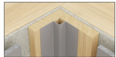
Bild 3 Swisspearl Inneneckprofil
