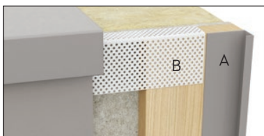
Bild 4 A. Swisspearl Plank Connect Abschlussprofil B. Swisspearl Lüftungsprofil
