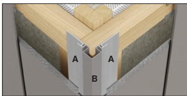
Bild 1 A. Swisspearl Plank Connect Anfangsprofil B. Swisspearl Außenecke klein
