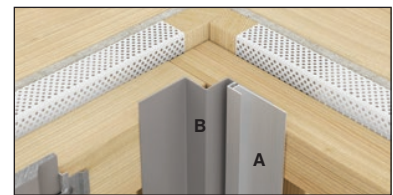
Bild 3 A. Swisspearl Plank Connect Anfangsprofil B. Swisspearl Außenecke klein
