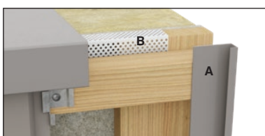
Bild 7 A. Swisspearl Plank Connect Abschlussprofil B. Swisspearl Lüftungprofil
