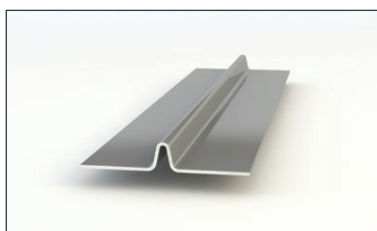
11. „Swisspearl“ v formos profilis 5x50 mm aliuminio profilis „nematomoms“ plokščių jungtims.
