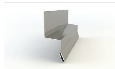
9. „Swisspearl“ nulašėjimo profilis, didelis 20x30x25 mm spalvoto aliuminio apdailos profilis.
