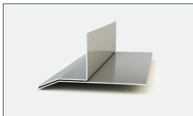
8. „Swisspearl“ horizontalus apdailos užbaigimo profilis, didelis 40x50x40 mm spalvoto aliuminio profilis užbaigimui virš durų ir langų.
