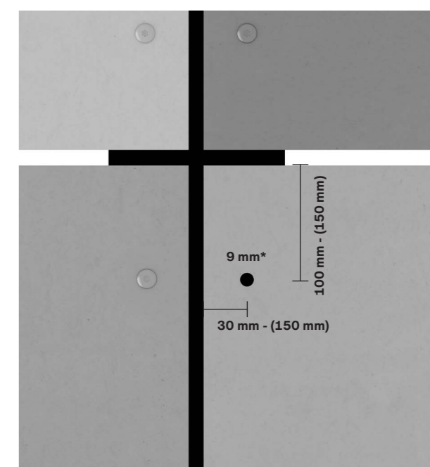
Kinnitite servakaugused
