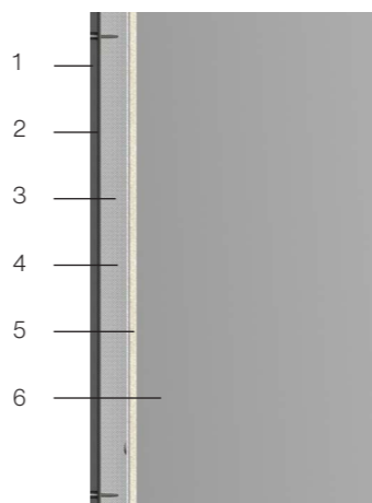
Liistuga tihendatud horisontaalvuuk
