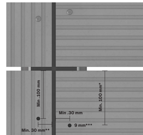
Pilt 3. Swisspearl Patina Inline plaadi paigaldamisel kasutatavad servakaugused NB! Minimaalne vahemaa või lähim järgmine hari ***9 mm puuritera neetidele
