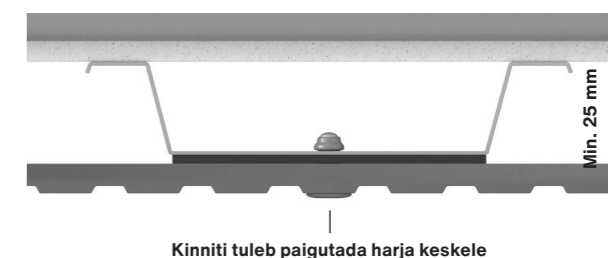
Pilt 2. Swisspearl Patina Inline plaadi paigaldamine keskmisele alusroovile
