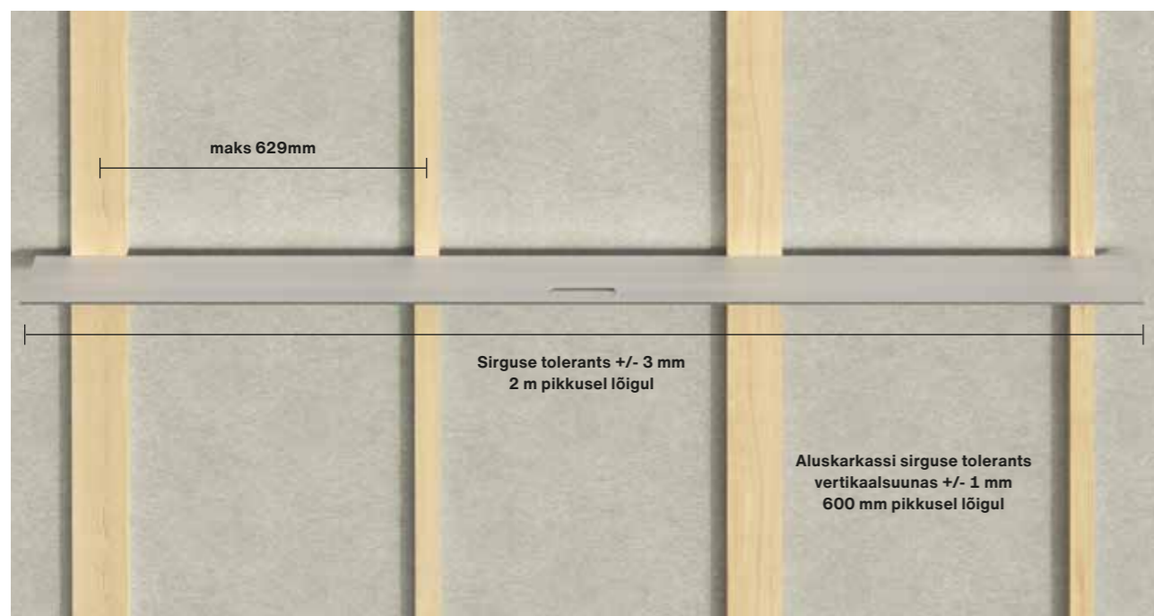
Aluskarkassi loodimine
