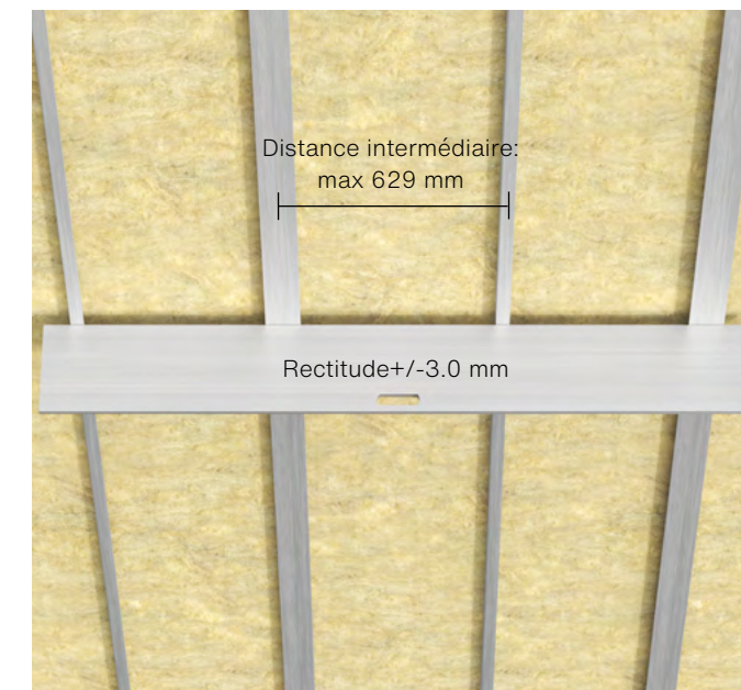
Rectitude de la construction sous-jacente
