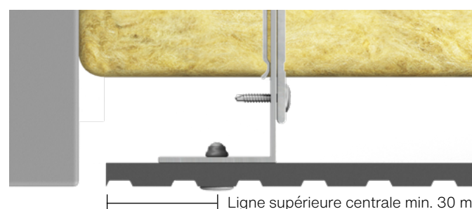
Fig. 4. Pose de panneaux Swisspearl Patina Inline sur panneau découpé sur mesure.
