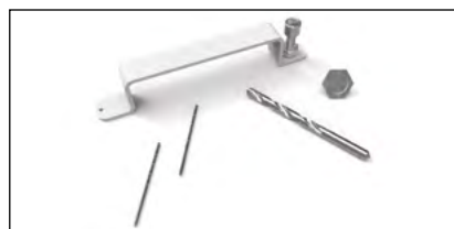
Kit d'outils aluminium 1. Outil de centrage pour aluminium 2. Tête de désolidarisation 3. 2 pièces. Forets HSS 4,1 mm 4. Foret TCT 9 mm
