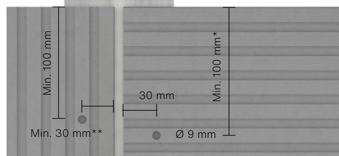
Fig. 3. Distance de fixation par rapport aux bords des panneaux Swisspearl Patina Inline.
